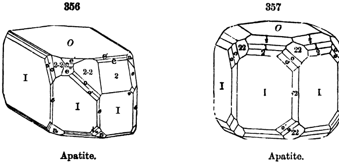
Apatite.
